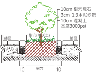
塊石樹穴剖面圖
