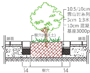
雪山岩樹穴剖面圖
