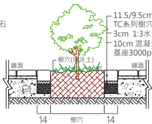
TC樹穴剖面圖
