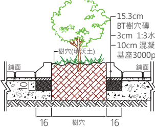
BT樹穴剖面圖
