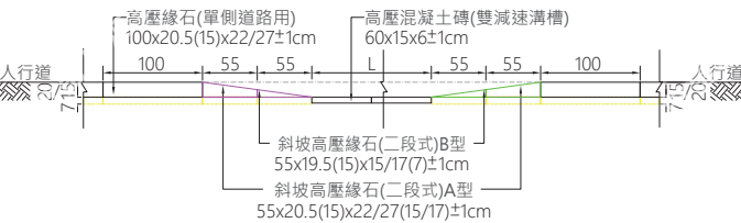
| H=22/27 二段式緣石無障礙斜坡道立面圖
