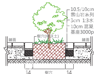
雪山岩樹穴剖面圖
