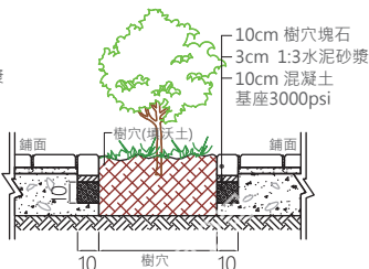
塊石樹穴剖面圖
