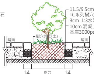
TC樹穴剖面圖
