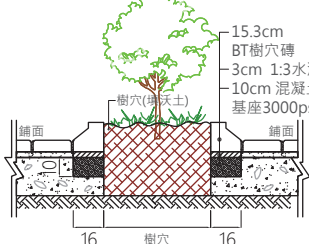
BT樹穴剖面圖
