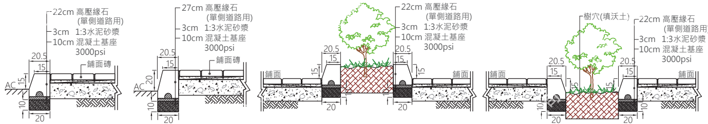
| H=22緣石收邊剖面圖 | H=27緣石收邊剖面圖 | H=22緣石(向外)樹穴剖面圖 | H=22緣石(向內)樹穴剖面圖
